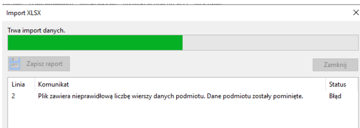
Rys. 20. Okno importu
